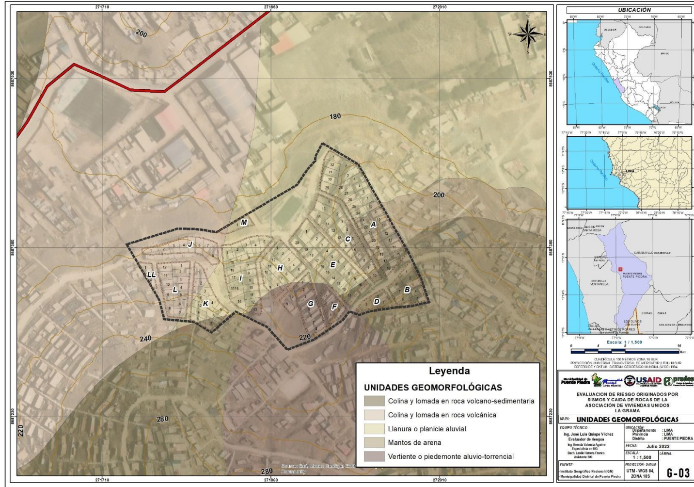
Mapa N° 9. Mapa Geomorfológico de la Asociación de Viviendas Unidos La Grama del distrito de Puente Piedra, provincia de Lima, departamento de Lima
